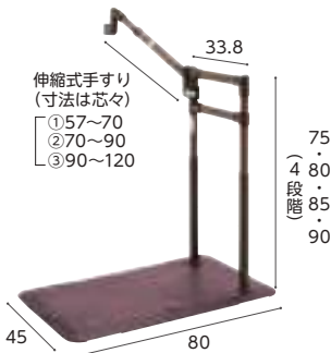
伸縮式手すり (寸法は芯々) ①57~70 ②70~90 ③90~120 重さ 約19.3kg 片手すり BZK-01S(N)
